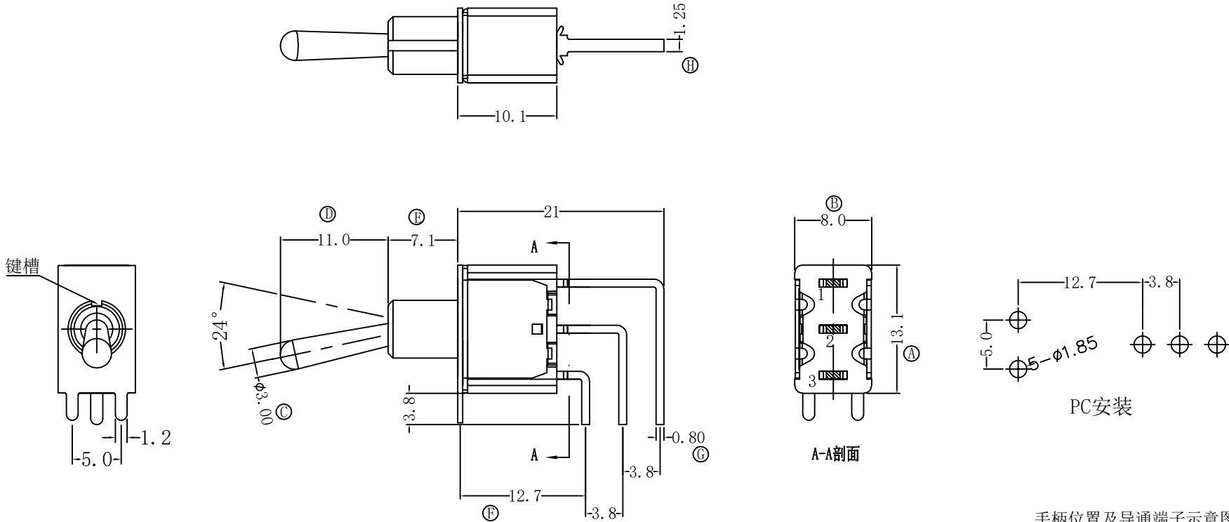
手柄位置及导通端子示意图
