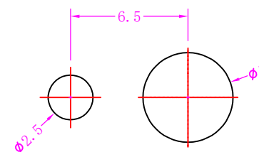
安装孔尺寸
