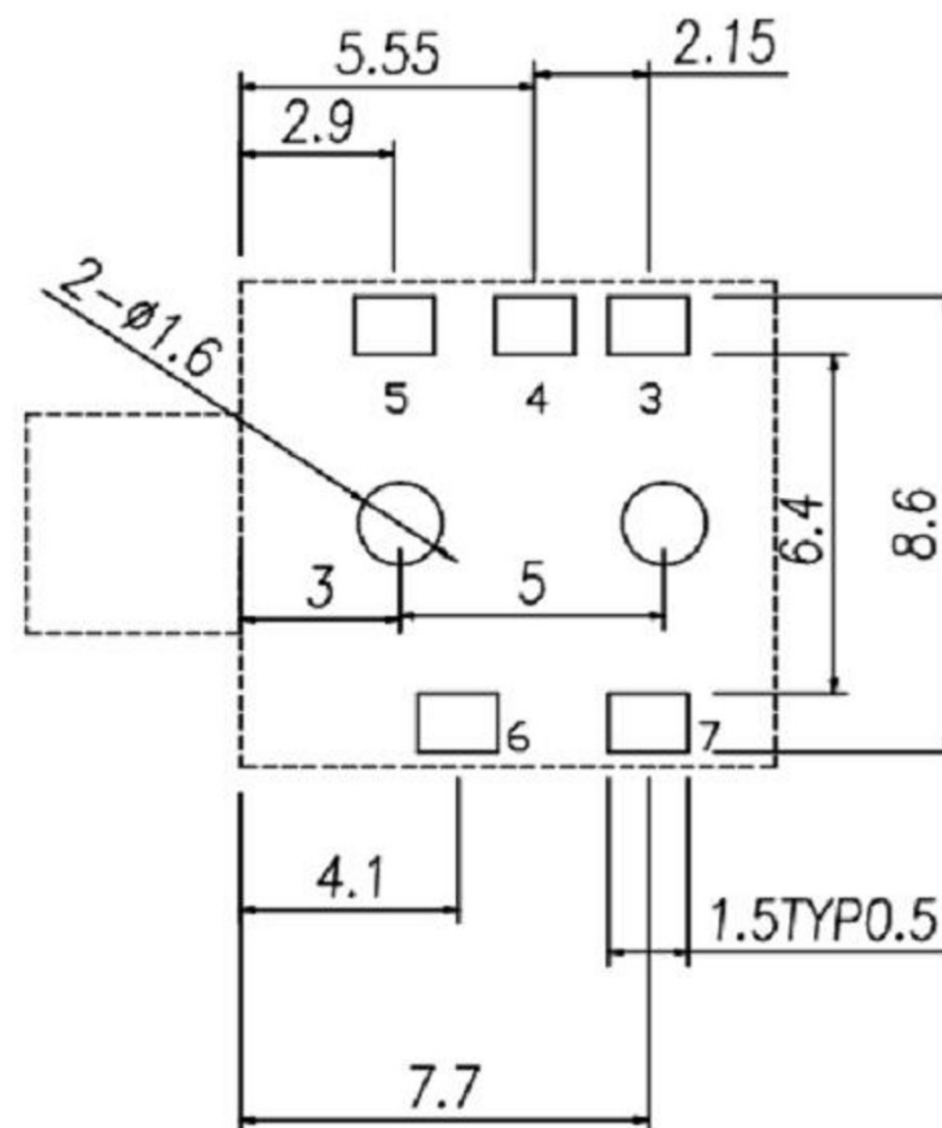
线路板安装尺寸示意图
