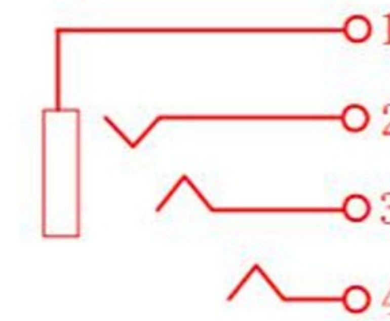
电路原理图
