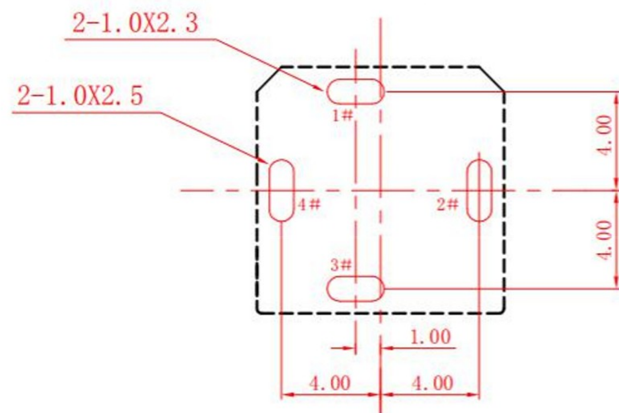
线路板开孔尺寸
