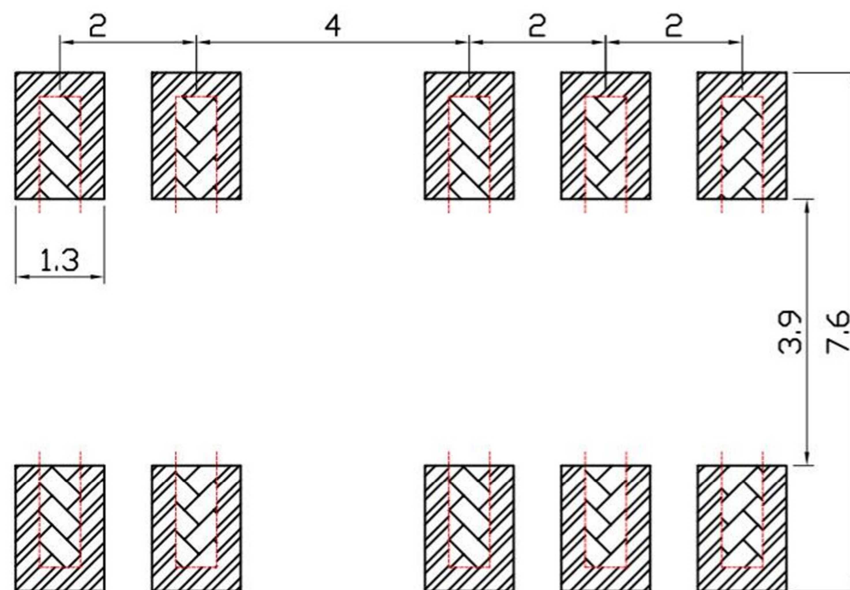
安装图 (PCB LAYOUT PLAN)
