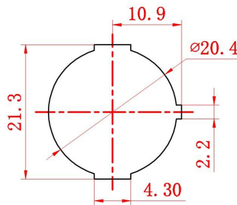
安装尺寸
