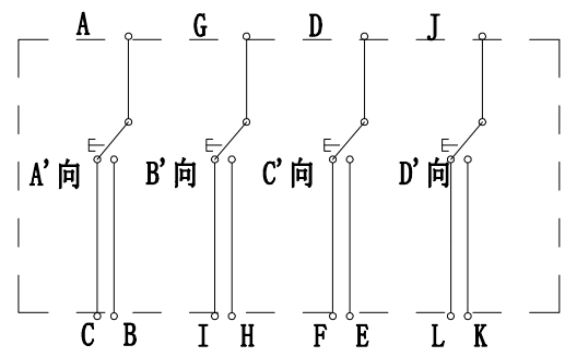
开关连接图
