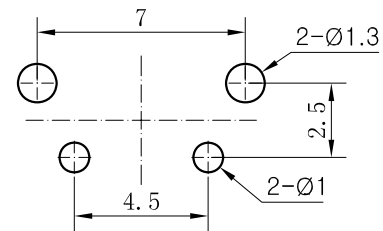
PCB线路板安装图(±0.1)
