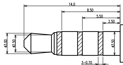
( \varnothing 3.5\text{mm} 4 POLE PLUG DETAIL DRAWING)
