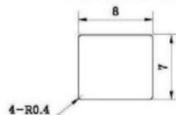
建议安装孔尺寸
