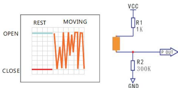
常用的电路接线方式
