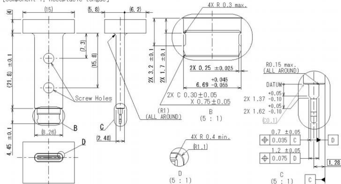
Receptacle tongue
