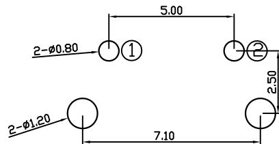
安装参考图
