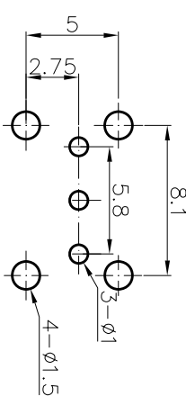
PCB线路板安装图(±0.1)
