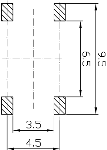
PCB线路板安装图(±0.1)
