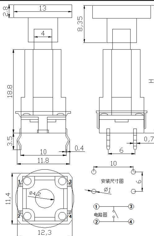
尺寸外型图
