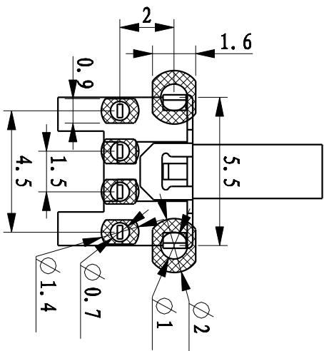
P.C.B LAYOUT
